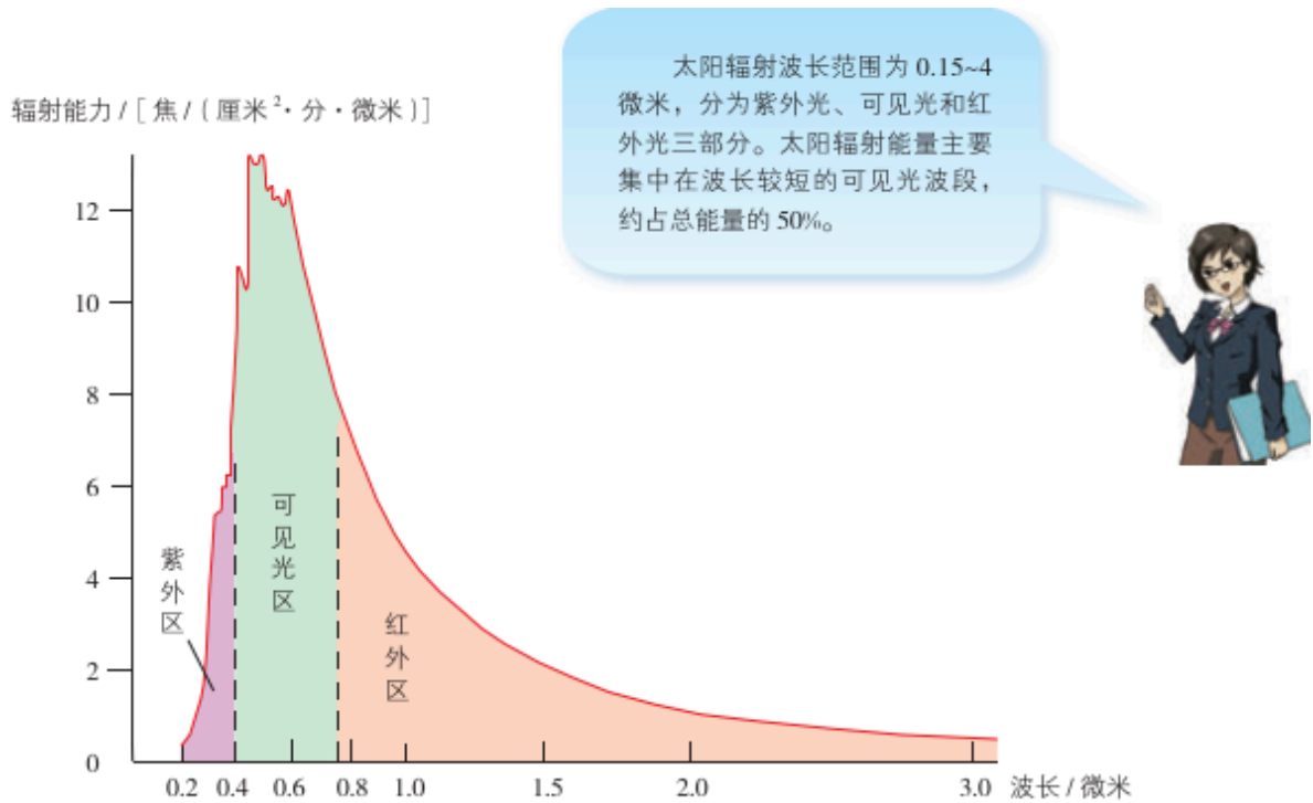
图 1-12 太阳辐射能量随波长的分布
