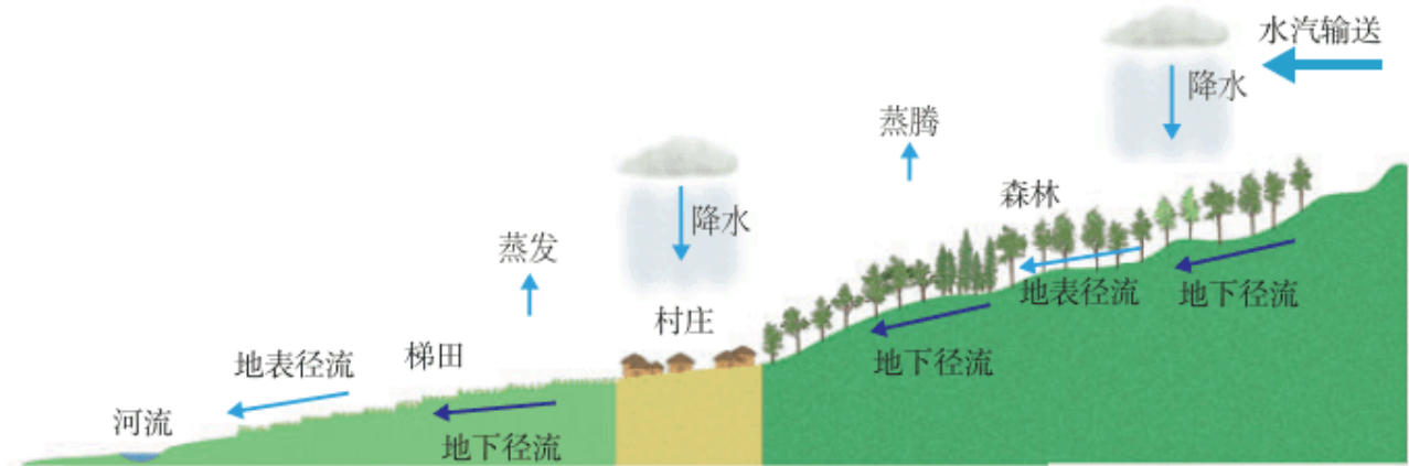
图 2.33 红河哈尼梯田景观及剖面示意
