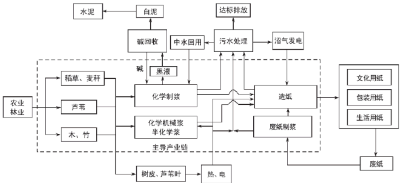
图1-5-6 某造纸企业绿色生产流程
