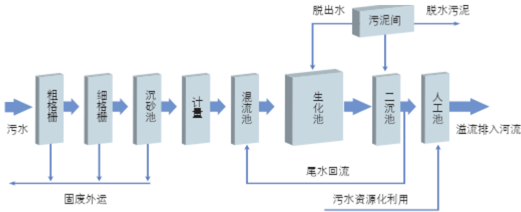
图 5-14 污水处理流程示意
