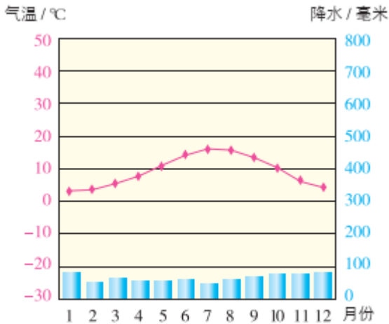
图 3-18 伦敦气温年变化曲线和逐月降水量
