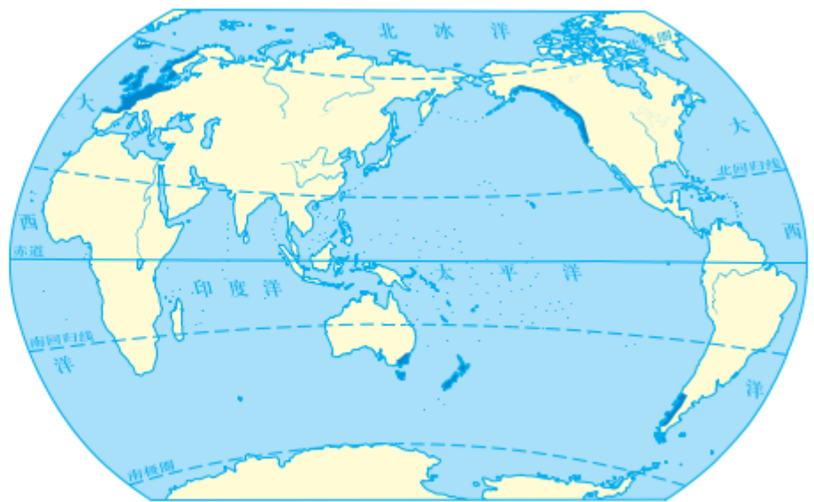
图 3-19 温带海洋性气候分布
