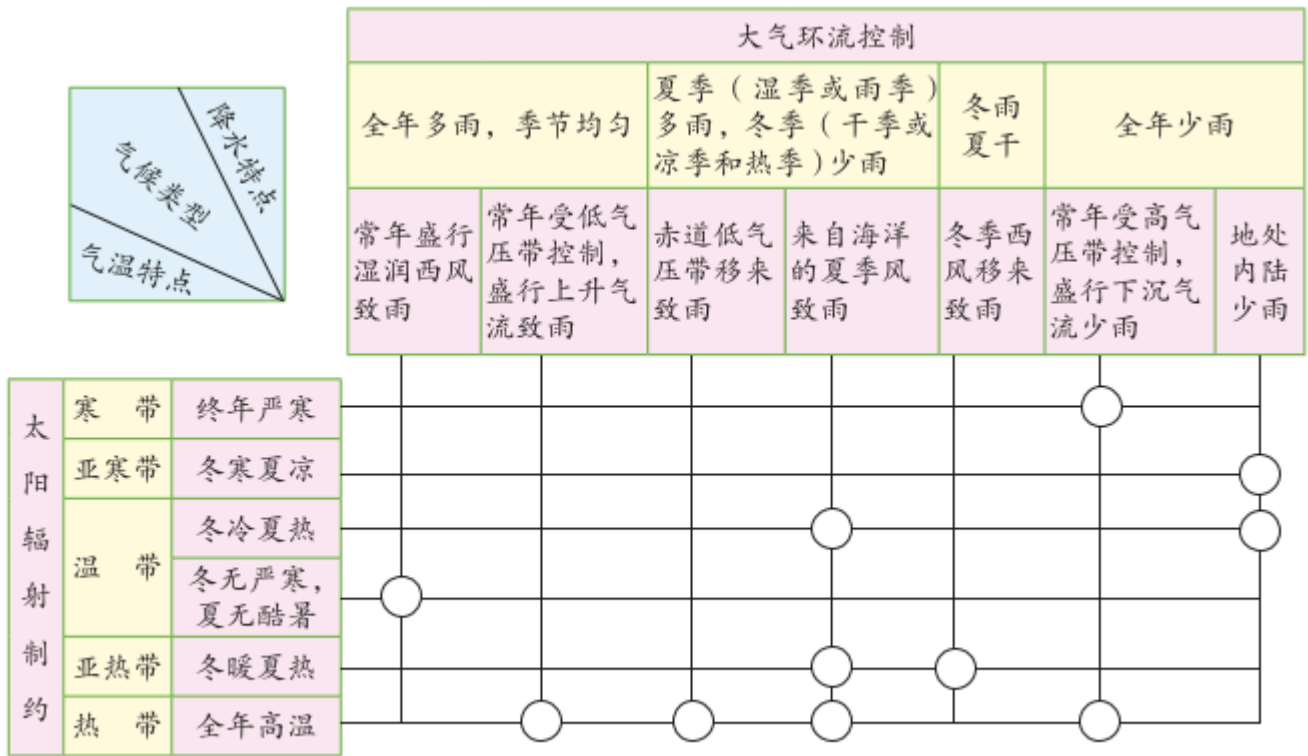
图 3-31 世界主要气候类型的形成原因
