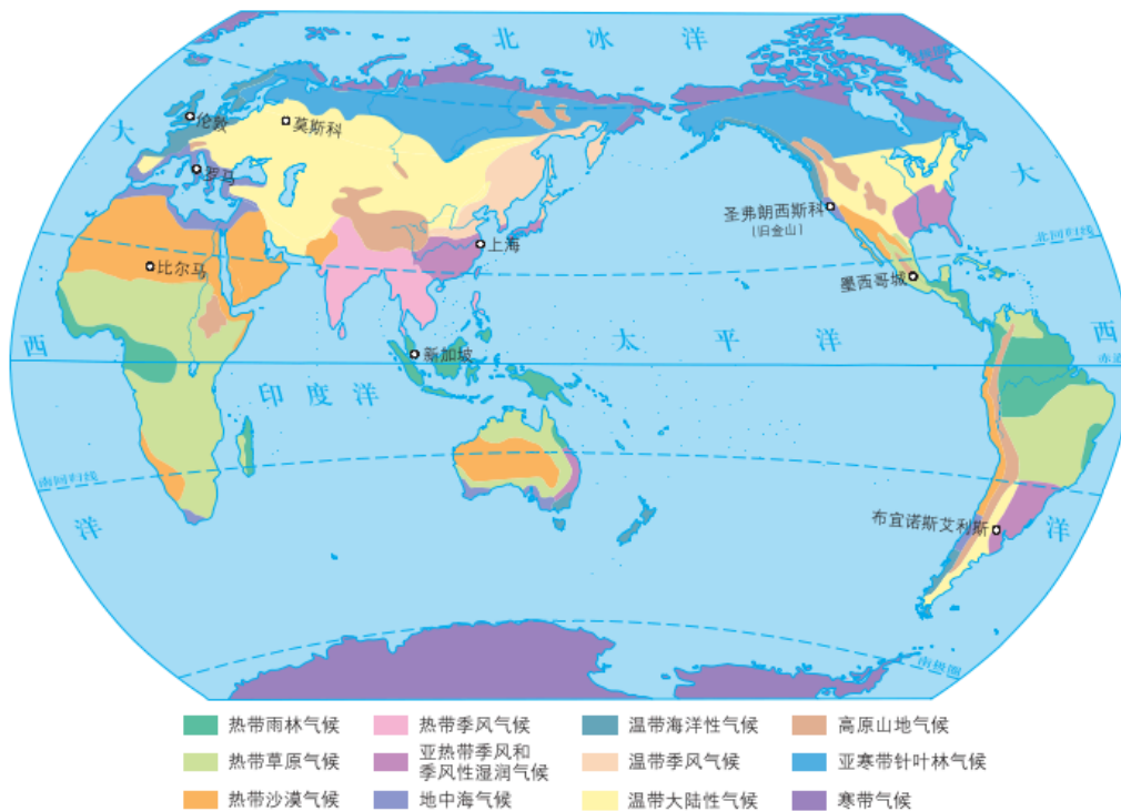
图 3-32 世界气候类型分布
