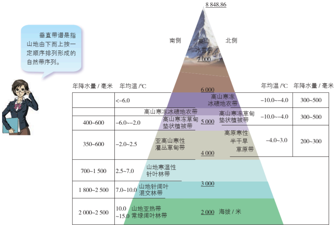
图 5-12 珠穆朗玛峰地区垂直自然带分布示意
