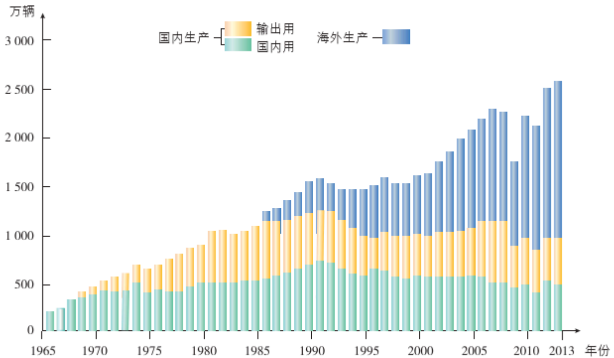
图 3-5 1965—2013 年日本汽车生产变化示意
